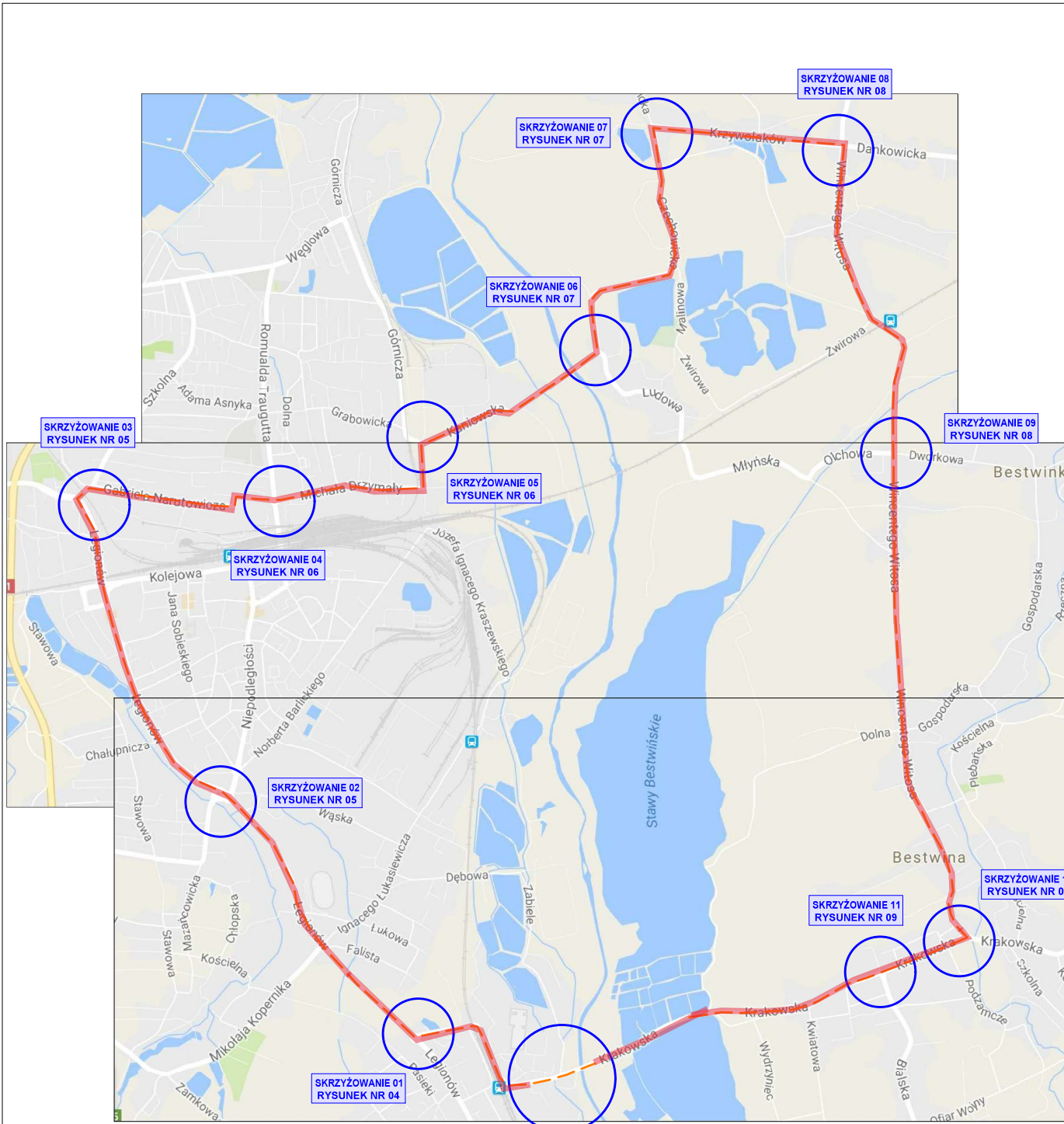
oznakowanie miejsca robót RYSUNEK NR 03
