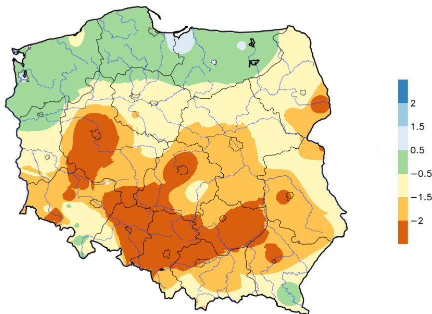
Rysunek 20 Rozkład przestrzenny wartości SPI na terenie kraju w czerwcu 2019 r.
