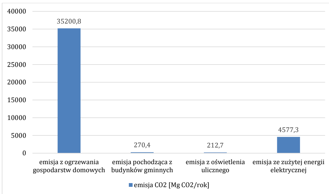
Rysunek 9 Emisja CO 2 z poszczególnych sektorów na terenie gminy Bestwina
